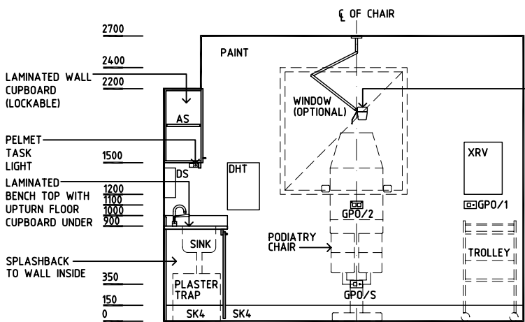
ELEVATION 1
