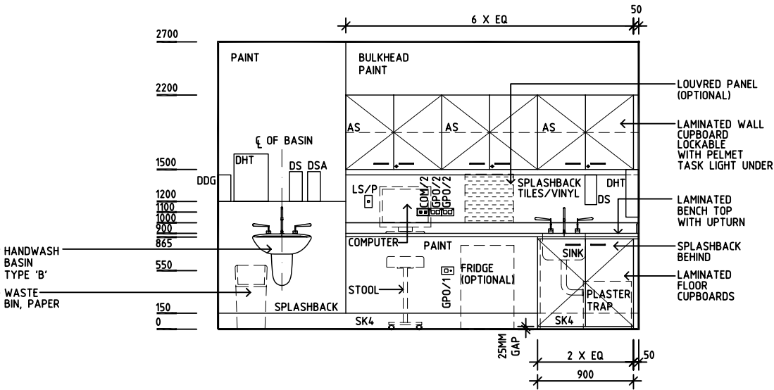
ELEVATION 4
