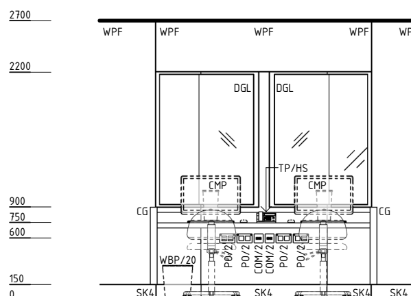
ELEVATION 1
