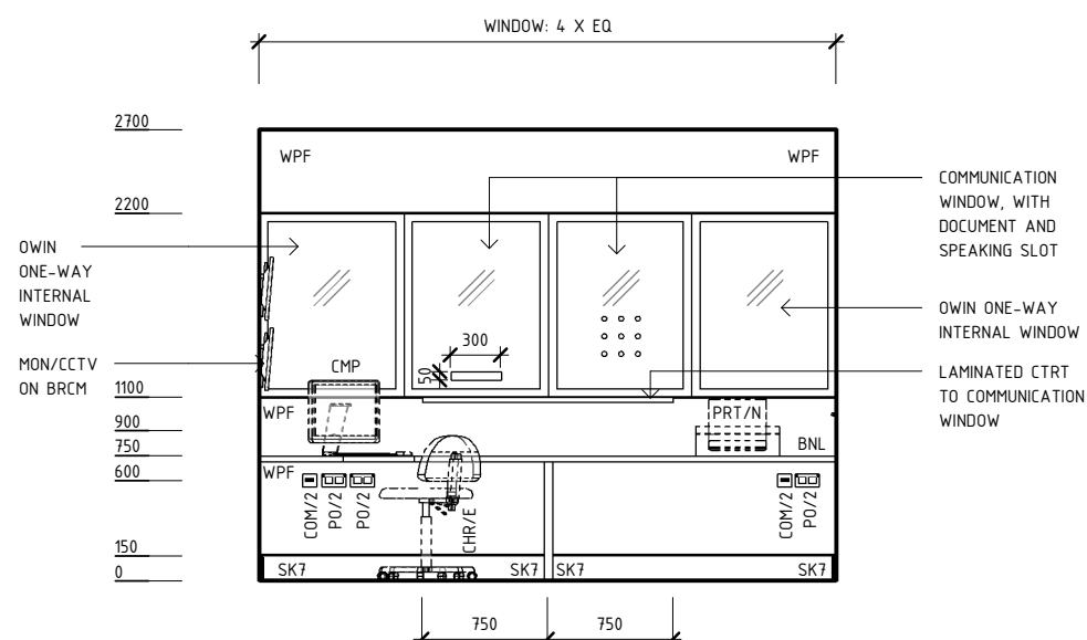
ELEVATION 2
