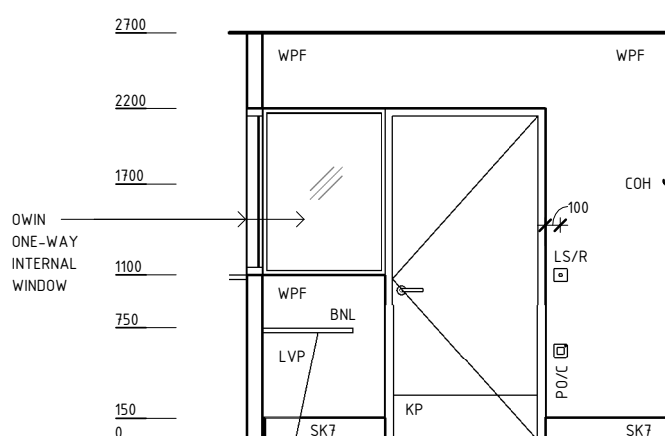
ELEVATION 3
