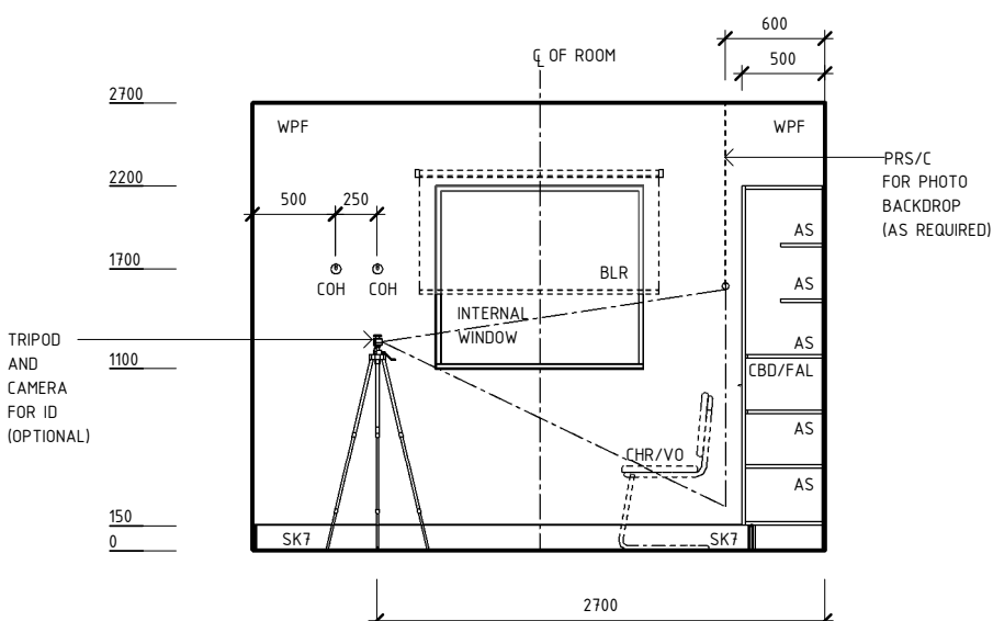
ELEVATION 4
