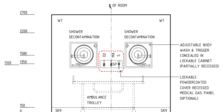
ELEVATION 2
