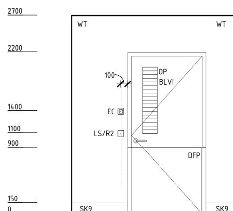
ELEVATION 3
