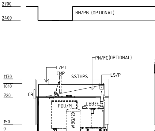
ELEVATION 3
