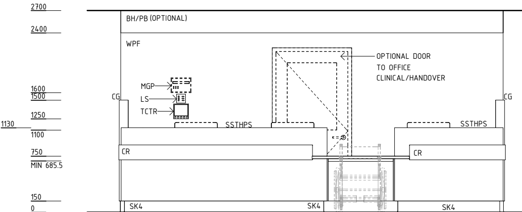
ELEVATION 2
