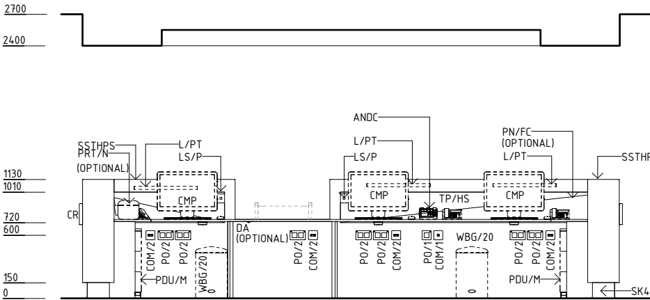
ELEVATION 5
