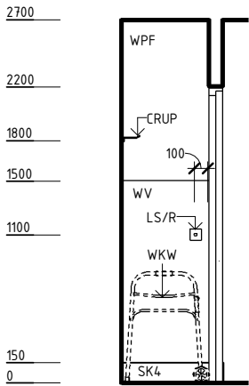
ELEVATION 2
