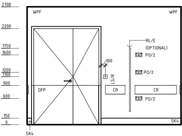
ELEVATION 3
