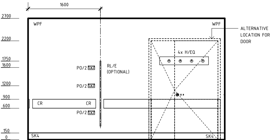
ELEVATION 2
