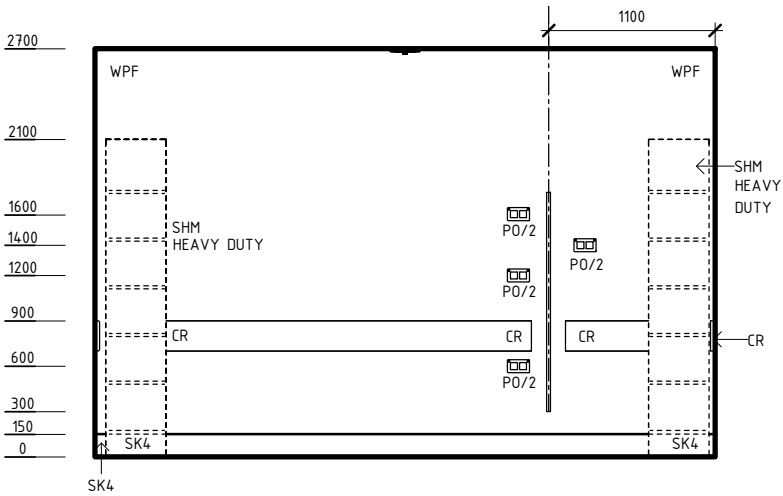
ELEVATION 1
