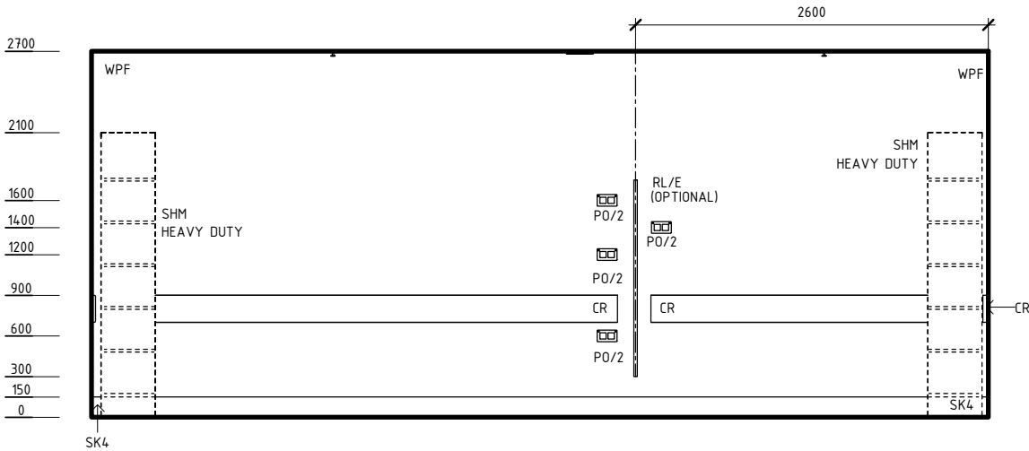
ELEVATION 1
