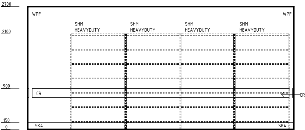
ELEVATION 4
