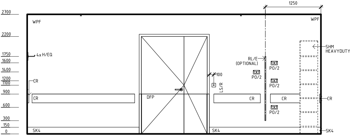
ELEVATION 3
