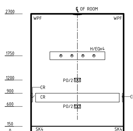
ELEVATION 2
