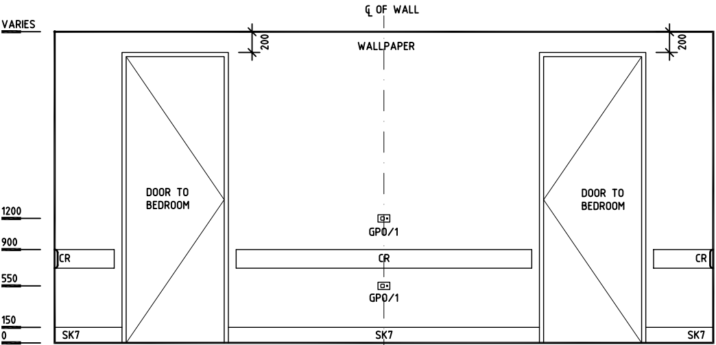
ELEVATION 4
