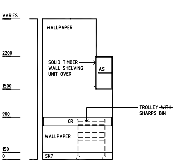
ELEVATION 1
