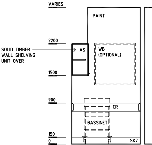
ELEVATION 3
