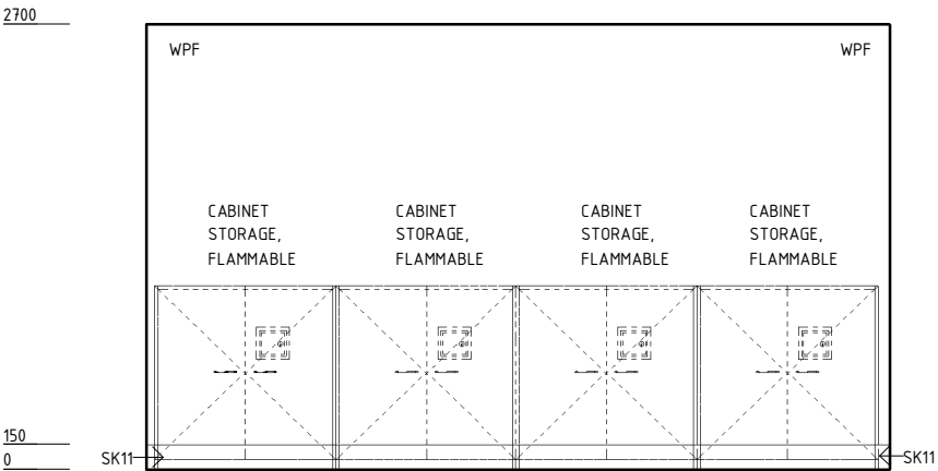
ELEVATION 2
