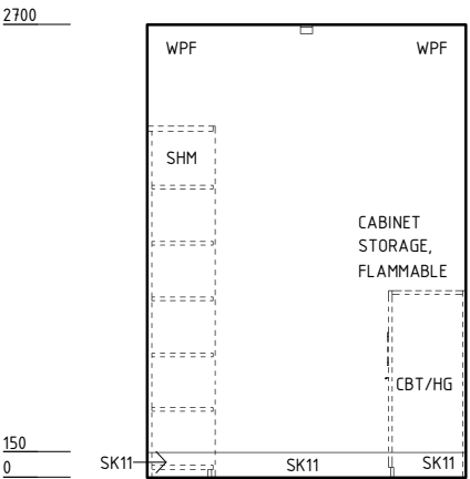
ELEVATION 1
