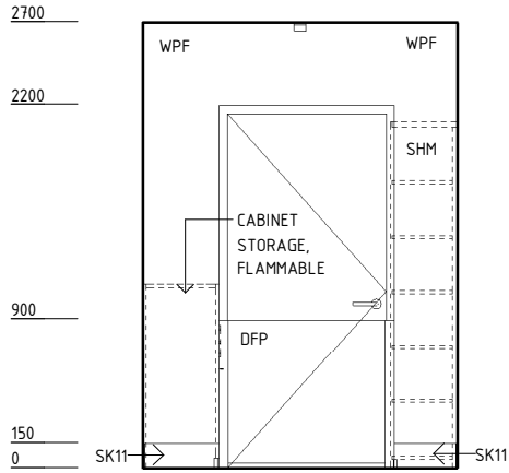
ELEVATION 3
