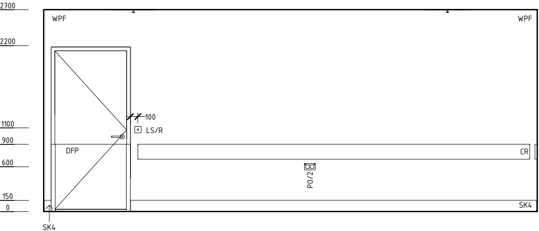
ELEVATION 3
