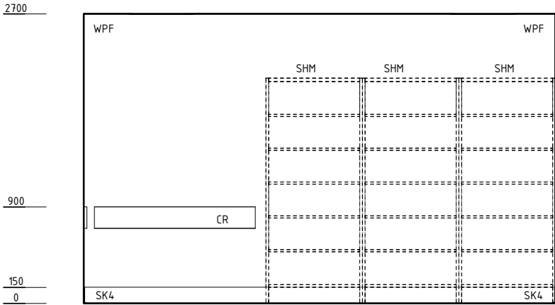
ELEVATION 4
