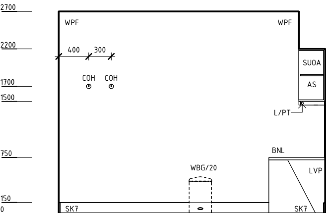
ELEVATION 4
