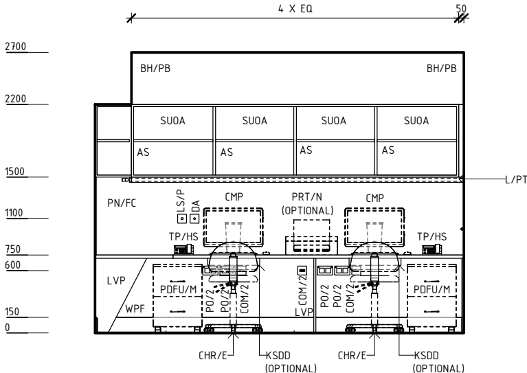
ELEVATION 2
