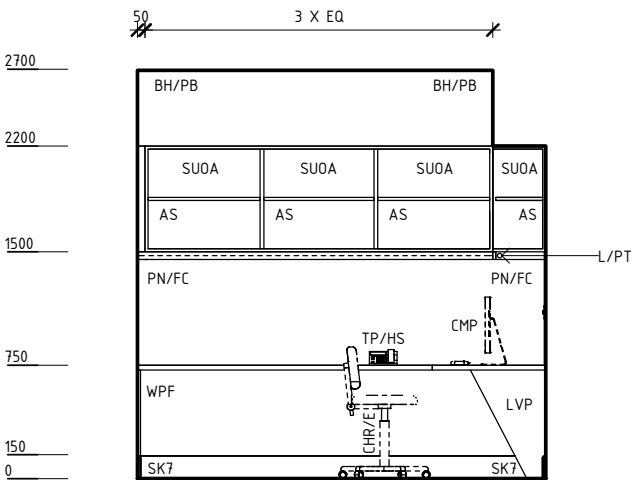
ELEVATION 1
