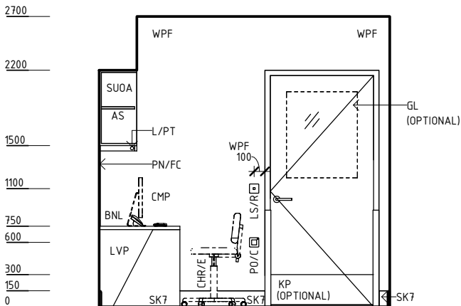
ELEVATION 3
