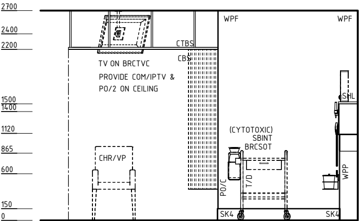
ELEVATION 2
