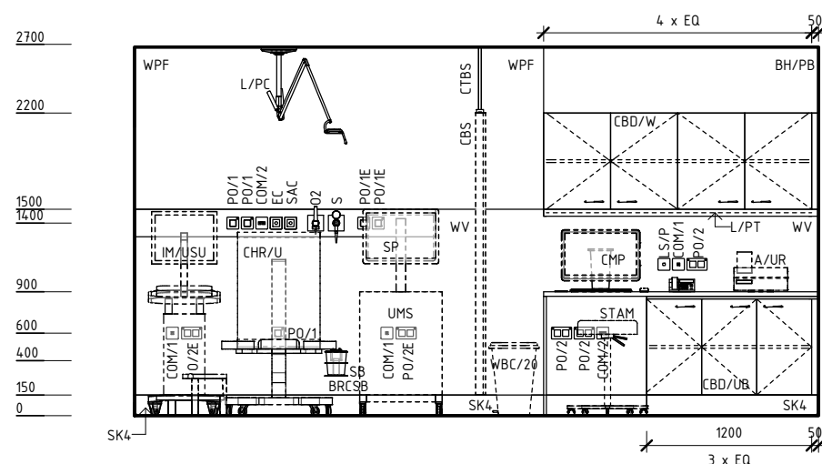
ELEVATION 2
