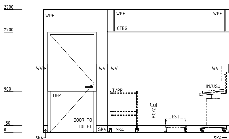
ELEVATION 1
