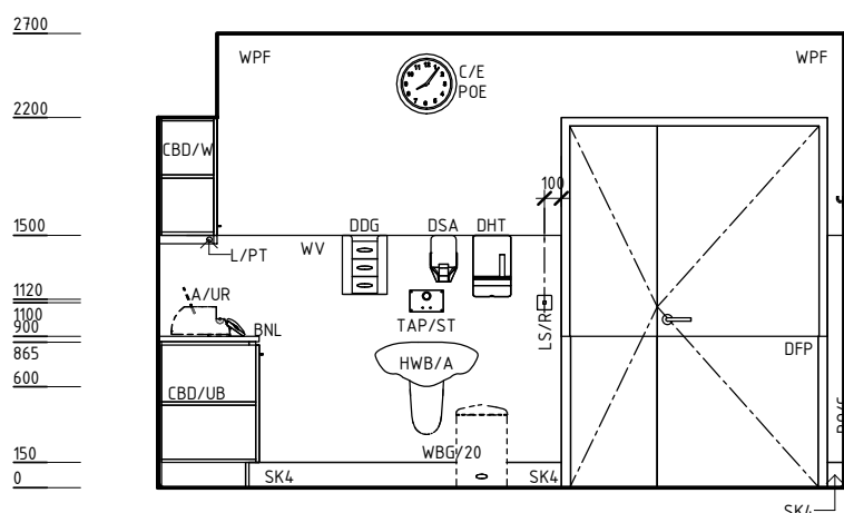
ELEVATION 3
