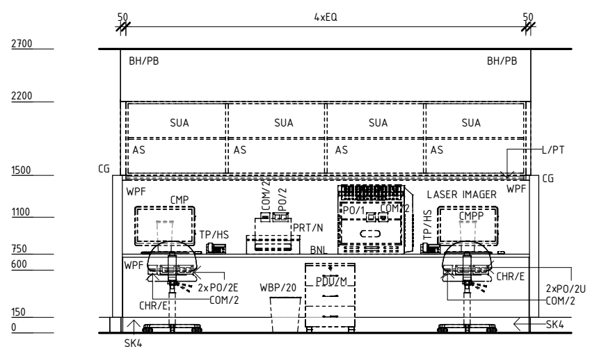
ELEVATION 2
