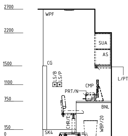
ELEVATION 1
