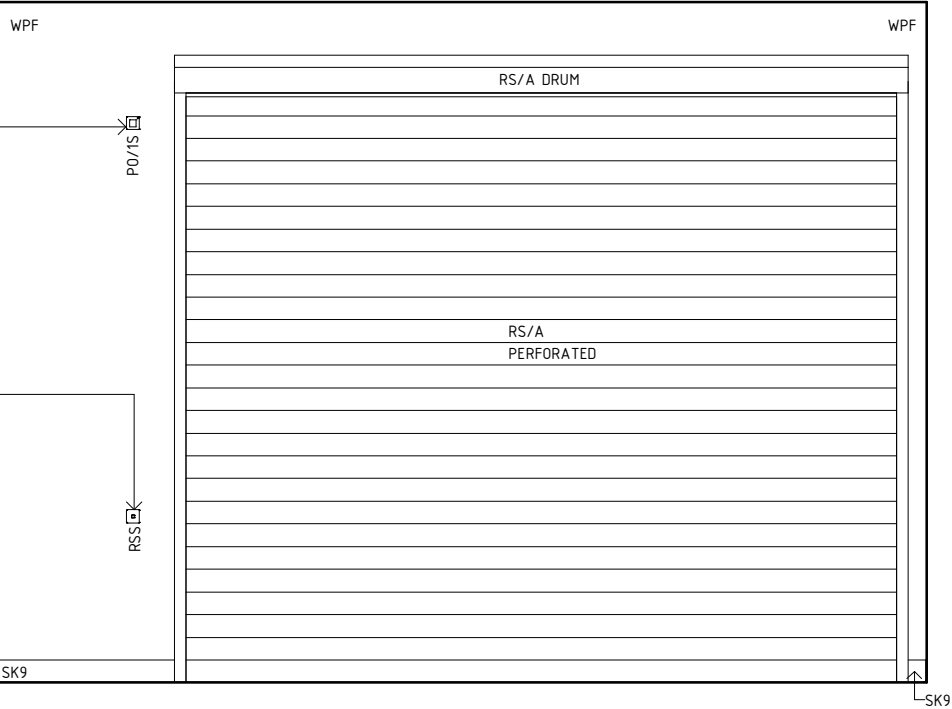
ELEVATION 3
