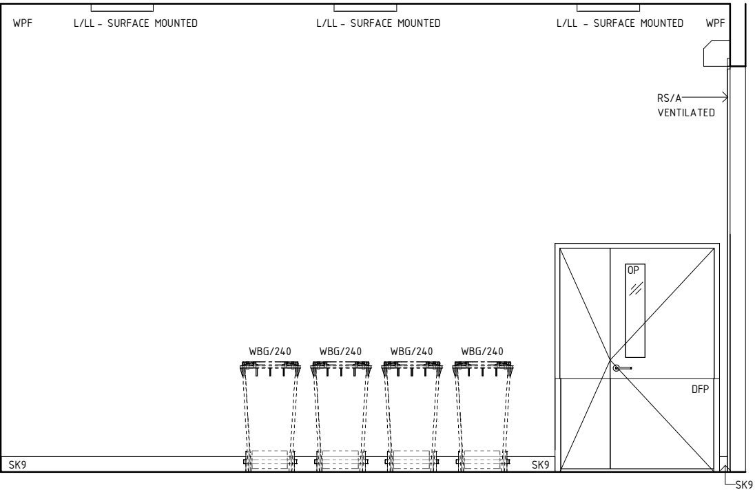
ELEVATION 2
