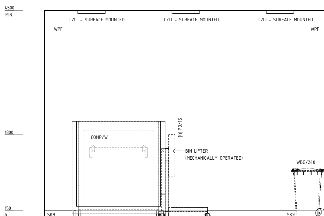
ELEVATION 1
