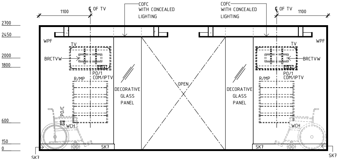
ELEVATION 3
