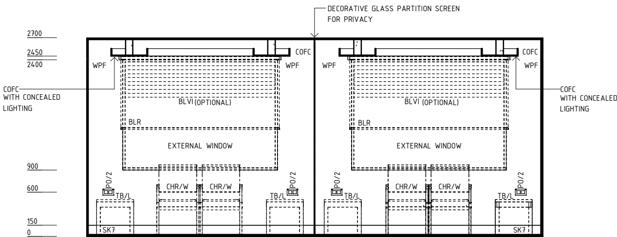
ELEVATION 1
