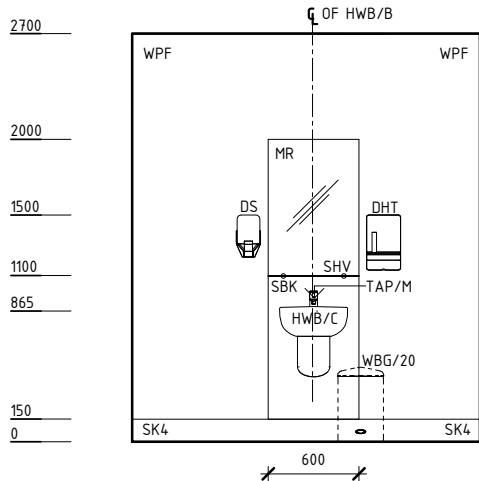
ELEVATION 4
