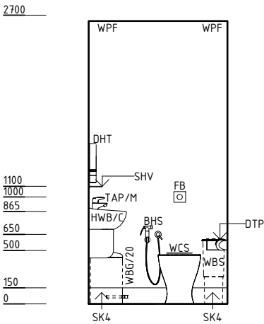
ELEVATION 1
