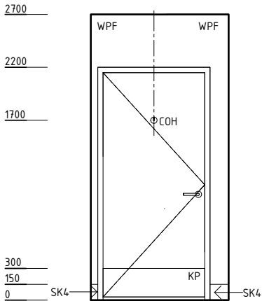
ELEVATION 3
