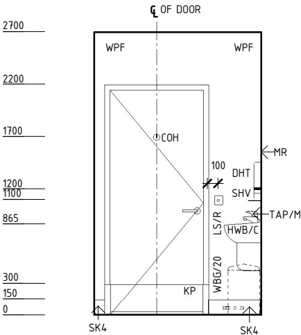
ELEVATION 3
