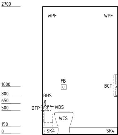
ELEVATION 1
