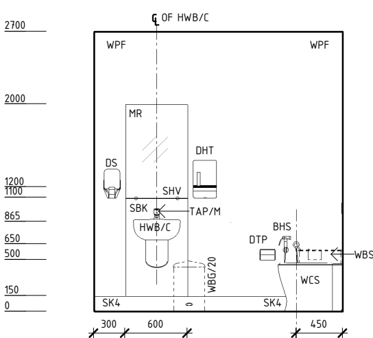
ELEVATION 4
