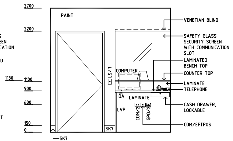
ELEVATION 2
