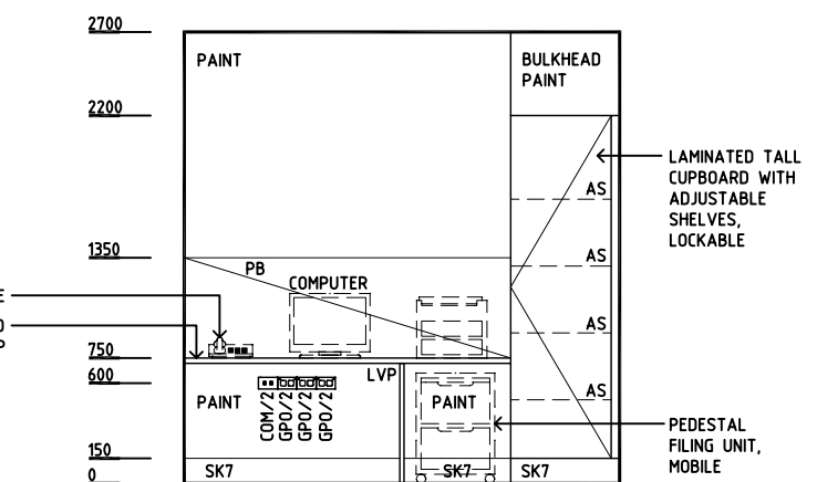
ELEVATION 4
