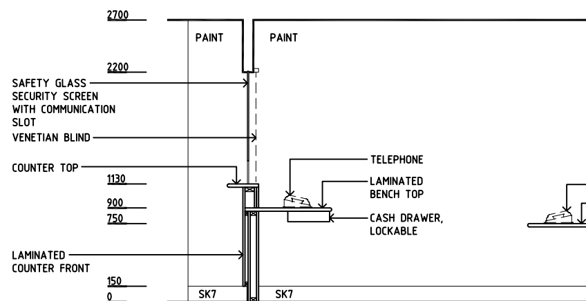
ELEVATION 3
