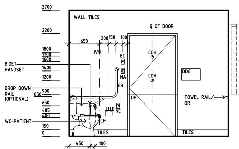
ELEVATION 1
