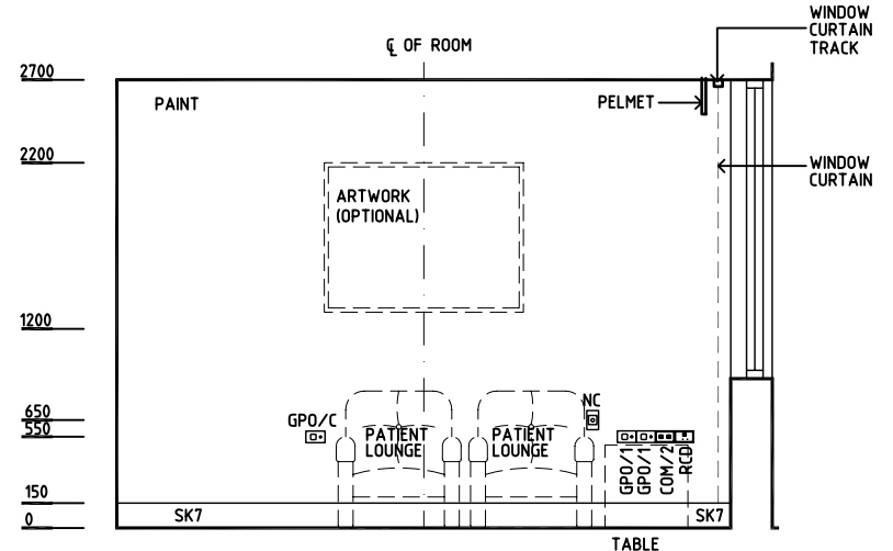
ELEVATION 4
