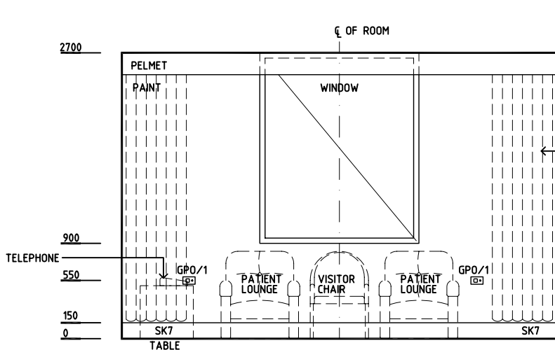
ELEVATION 1
