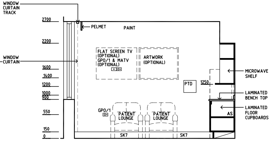
ELEVATION 2
