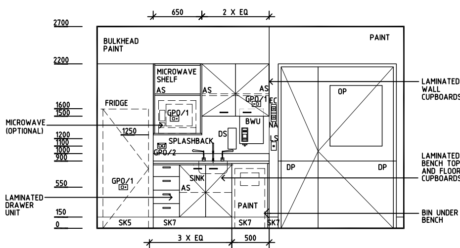
ELEVATION 3
