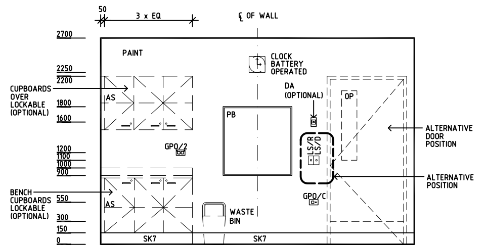
ELEVATION 2
