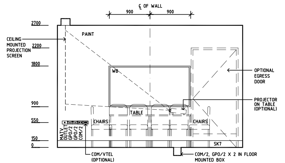
ELEVATION 4
