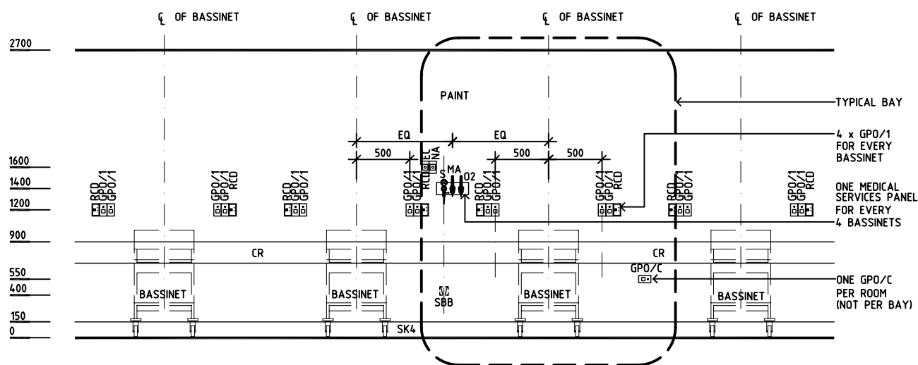
ELEVATION 1
