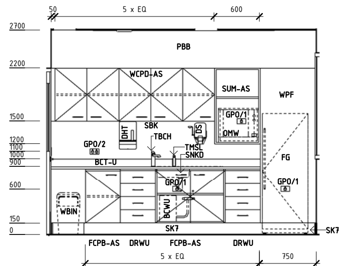
ELEVATION 4
