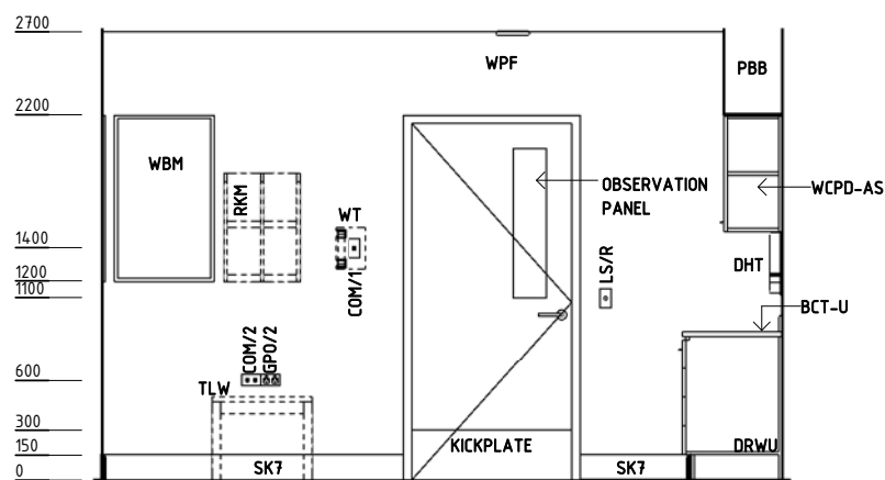
ELEVATION 3
