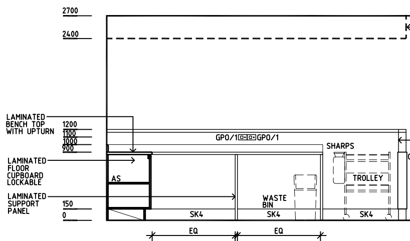
ELEVATION 3
