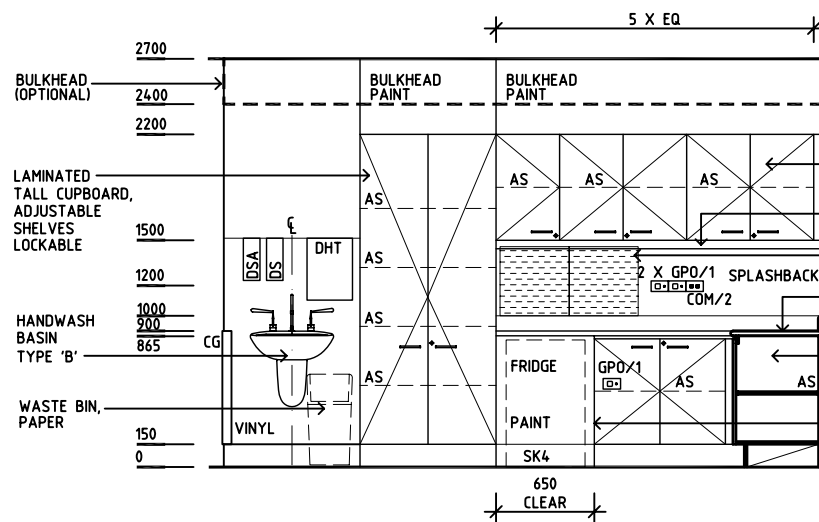
ELEVATION 1
