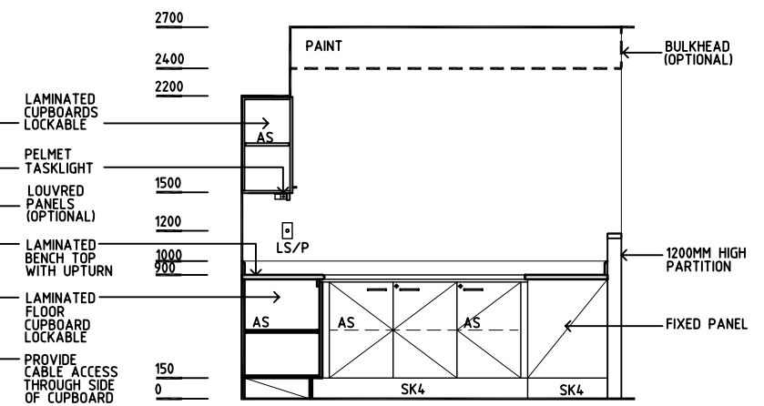
ELEVATION 2
