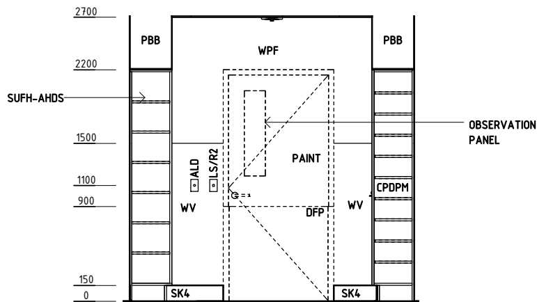
ELEVATION 1
