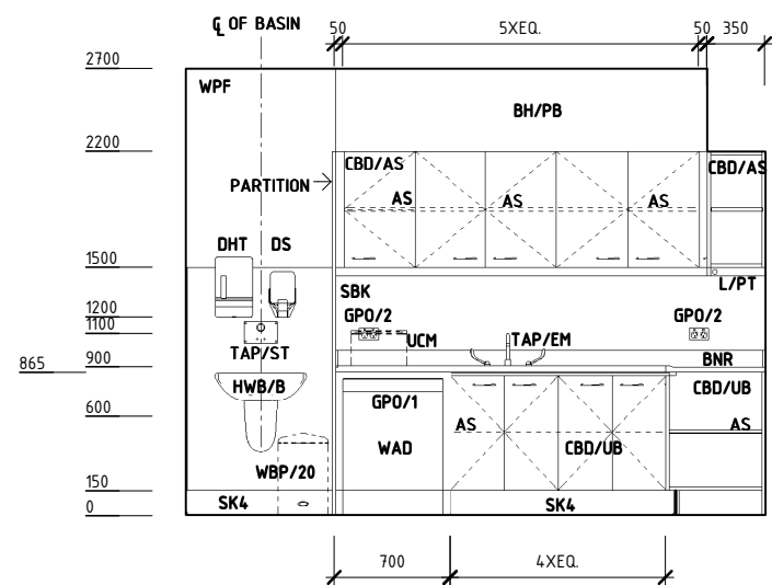
ELEVATION 4
