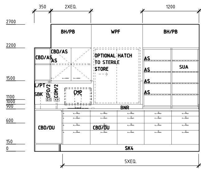
ELEVATION 2
