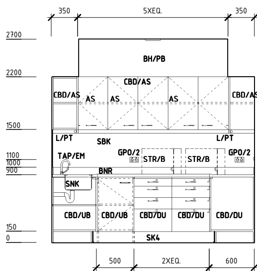
ELEVATION 1
