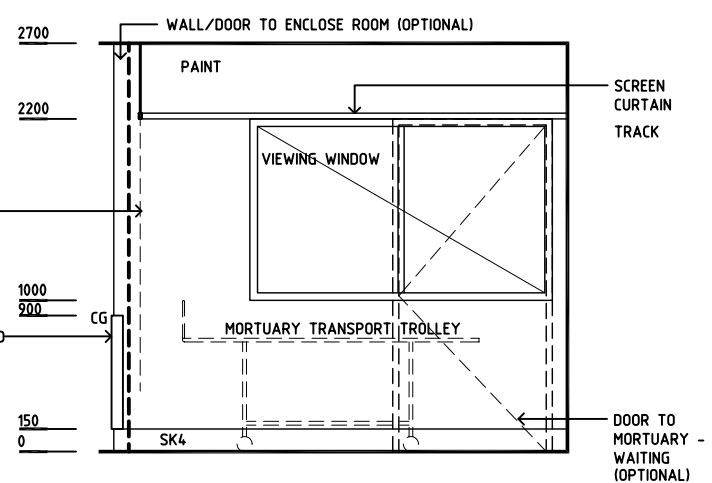
ELEVATION 4
