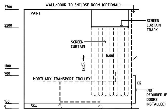
ELEVATION 2
