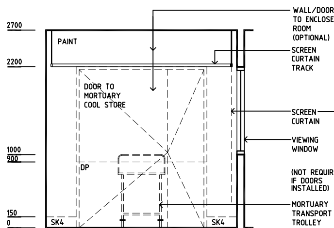
ELEVATION 3
