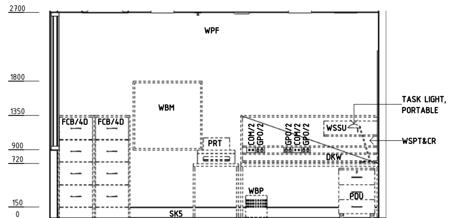
ELEVATION 2
