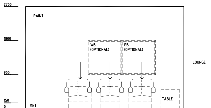
ELEVATION 4
