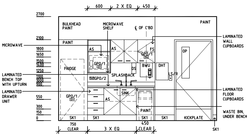
ELEVATION 3
